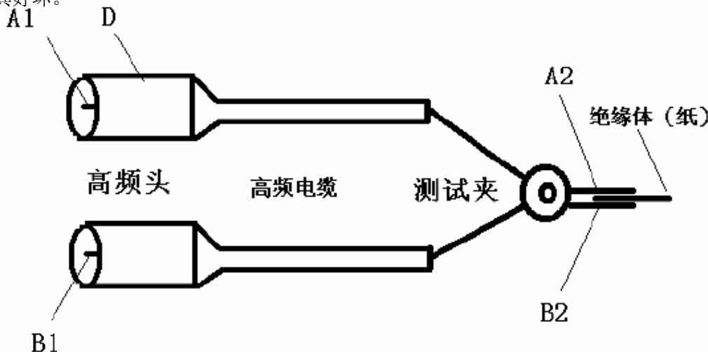
图 9-1 测试电缆局部连线图
