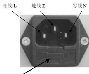
图 3-2 保险丝座 (随机附有两个保险丝)
