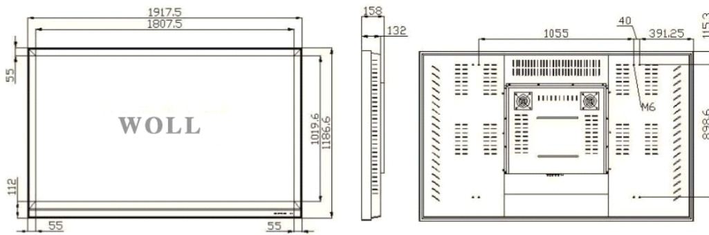
正视图
