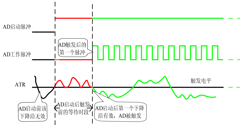
5.3 下降沿触发图例
