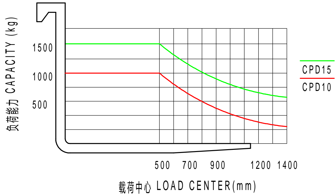
负荷曲线图 LOAD CURVE
