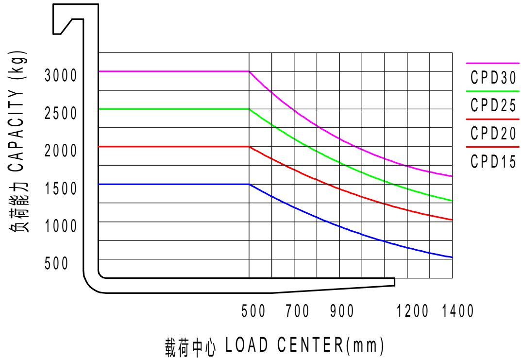
负荷曲线图 LOAD CURVE
