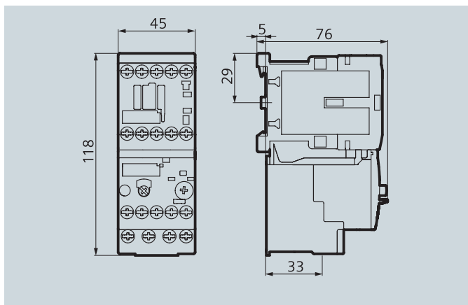
3RU21 16 S00 规格, 插接于 3RT2 接触器, 螺钉接线端子
