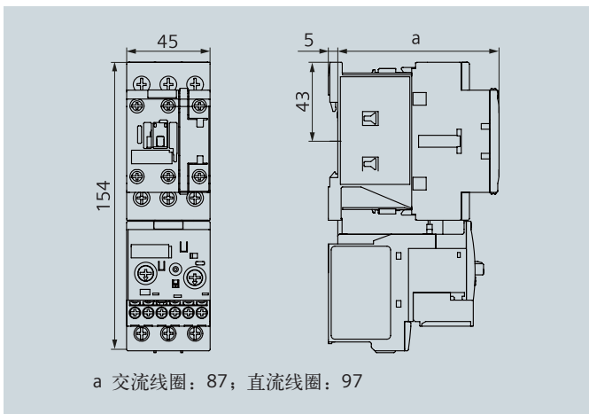
3RB3.2-..B0
