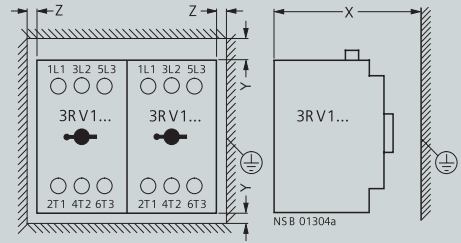
断路器和接地之间的间隙
