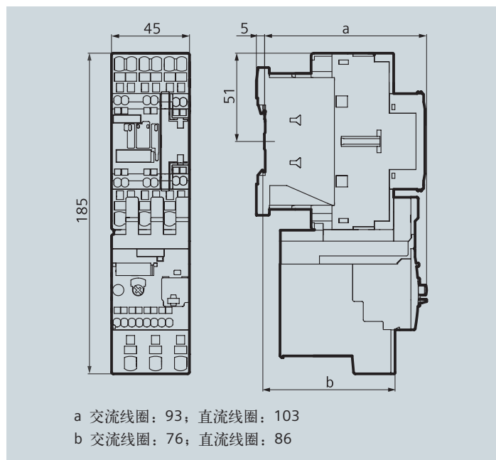
3RU21 26 S0 规格, 插接于 3RT2 接触器, 弹簧式接线端子
