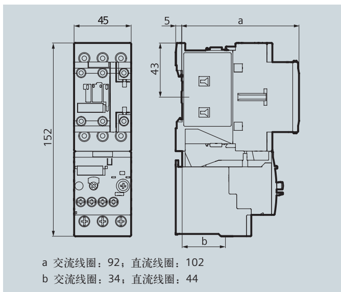
3RU21 26 S0 规格, 插接于 3RT2 接触器, 螺钉接线端子
