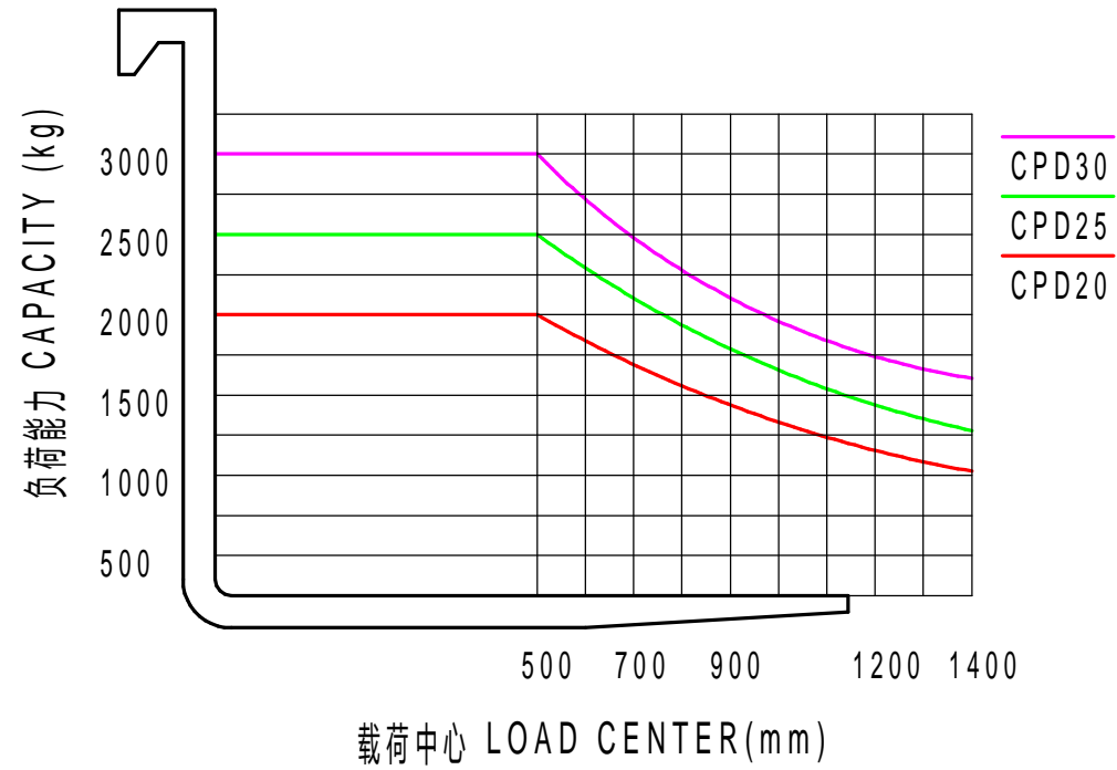
负荷曲线图 LOAD CURVE
