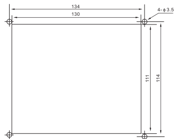
BK2E双电源控制器开孔图 总深度73mm, 安装柜体内深度61mm 用4-M3x10自攻螺丝固定
