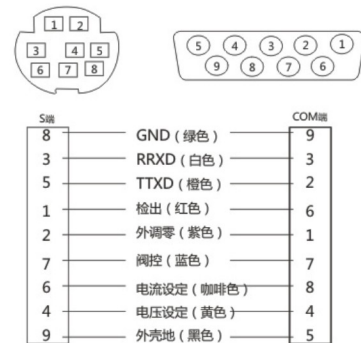
S端子与D-600CD/MD接线图
