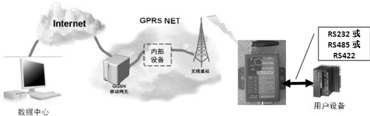
连接好的DTU系统
