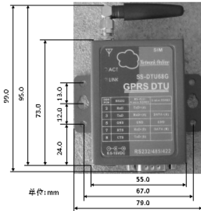
图 2.2 SS-DTU68G 外壳机械尺寸图
