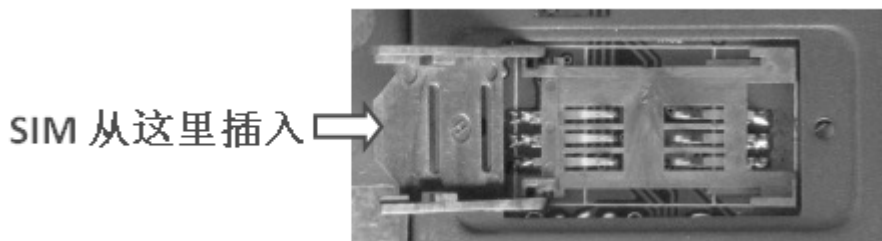
图2 SIM 卡的安装
