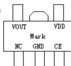
SOT-89-5
