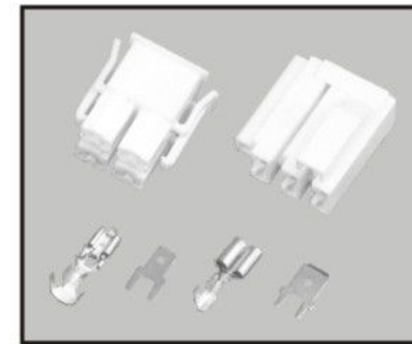
(4.8带锁/6.3轻插) 洗衣机系列
