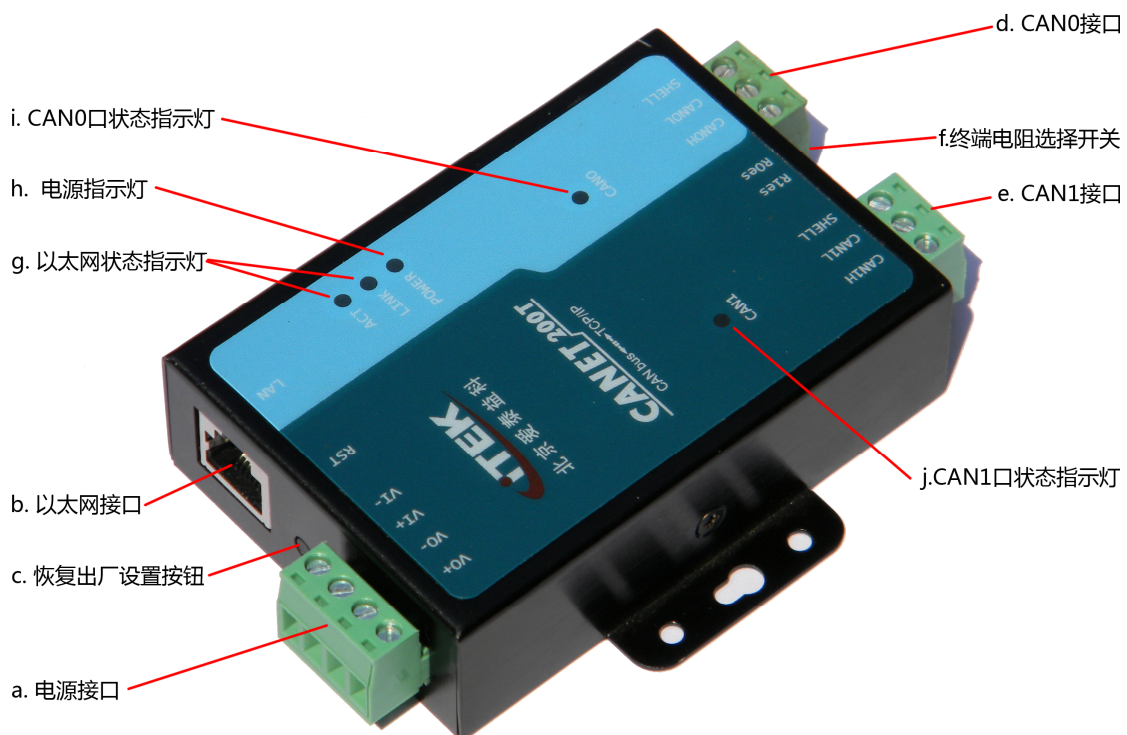
图 2.1 CANET-200T 外观图
