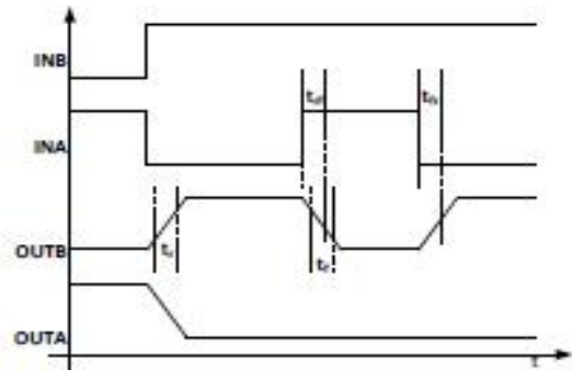
时间参数定义
