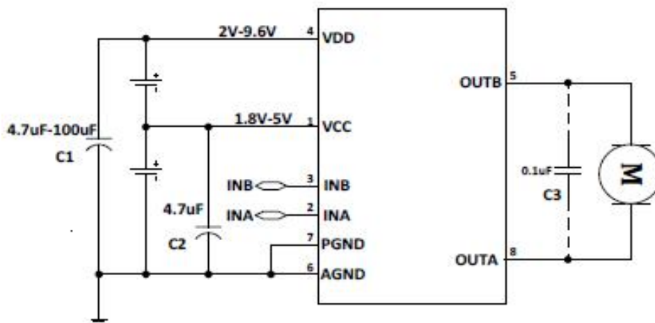
图 1 MX608 典型应用线路图
