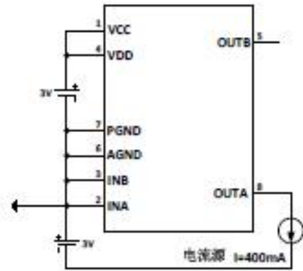
NMOS 体二极管导通电压测试原理图
