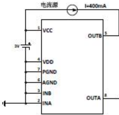
PMOS 体二极管导通电压测试原理图
