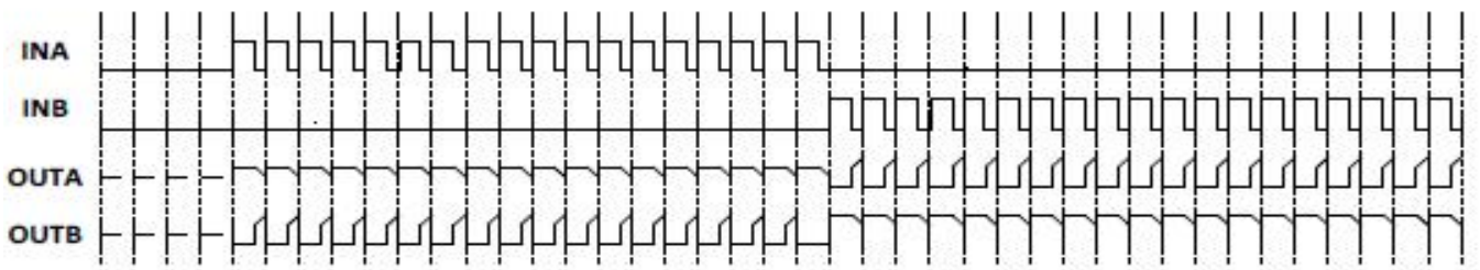
PWM 模式 A 信号波形示意图
