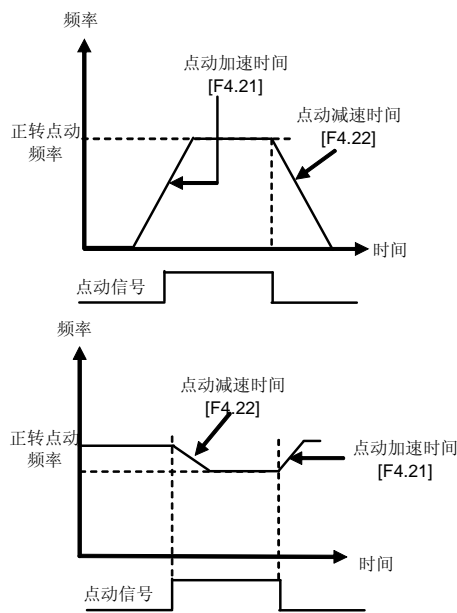
图 6-19 点动运行
