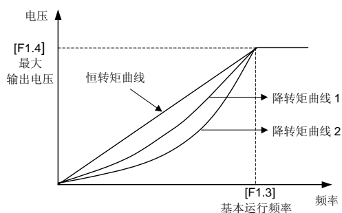
图 6-4 V/F 曲线
