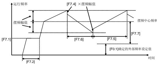
6-27 摆频运行过程
