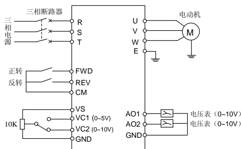
图 10-2 基本接线图
