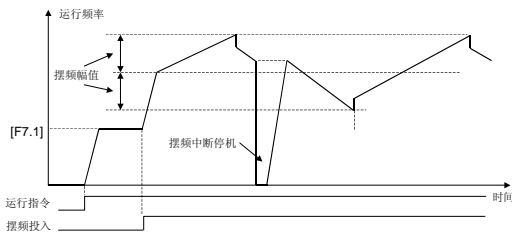
6-28 断点记忆恢复（条件有效方式）
