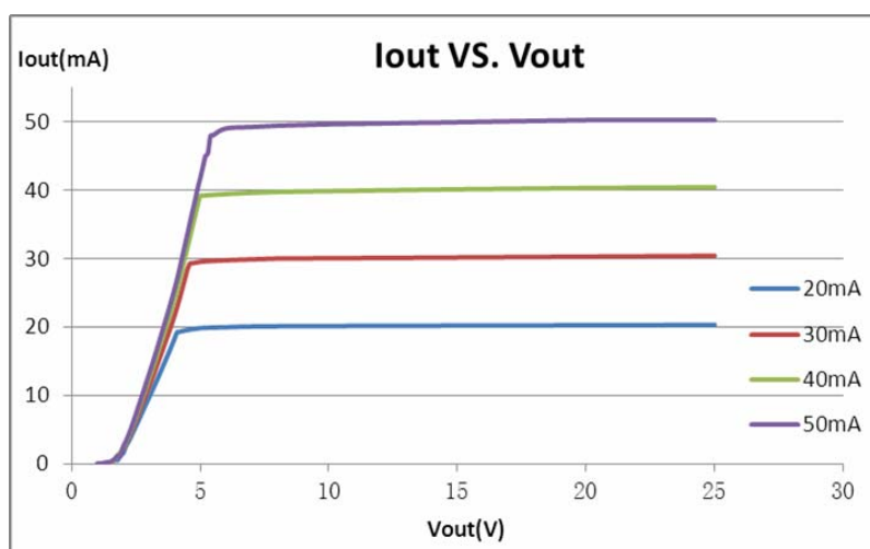
图 4. SM2082B 恒流曲线图
