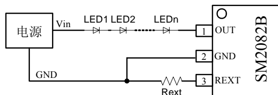
图 6. SM2082B 应用电路原理图
