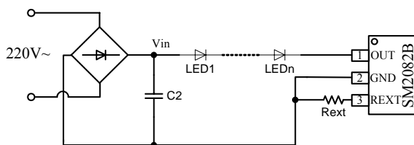
图 2. SM2082B 典型应用电路
