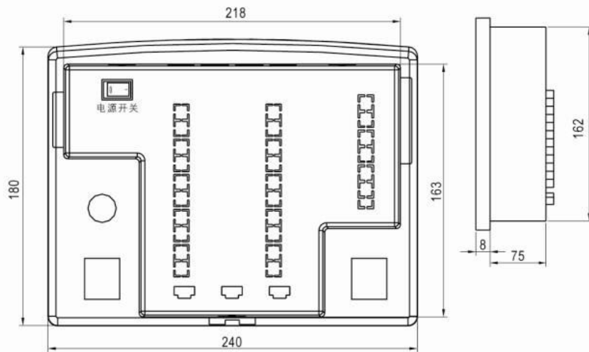
尺寸图(单位mm)
