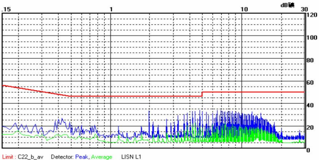
WRA2415P-3WR2 外围状态下电源正极 (Class B) 测试结果
