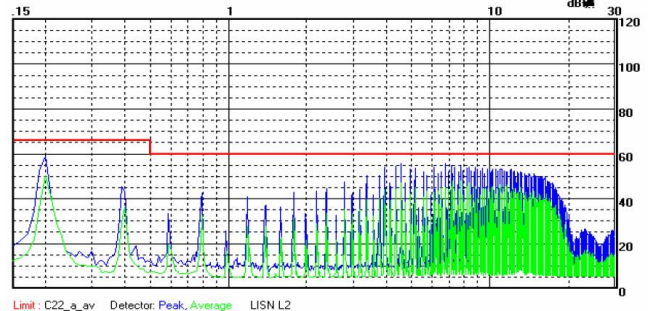
WRA2415P-3WR2 裸机状态下电源负极 (Class A) 测试结果
