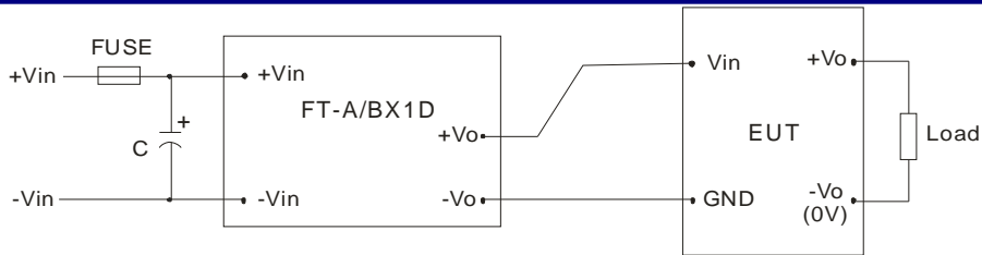
标称输入电压小于 48V 时, C \geq 330\mu\text{F}/50\text{V} 标称输入电压等于 48V 时, C \geq 330\mu\text{F}/100\text{V} FT-A/BX1D 为我司脉冲群抑制器, 具体型号请参照选型手册 图 3
