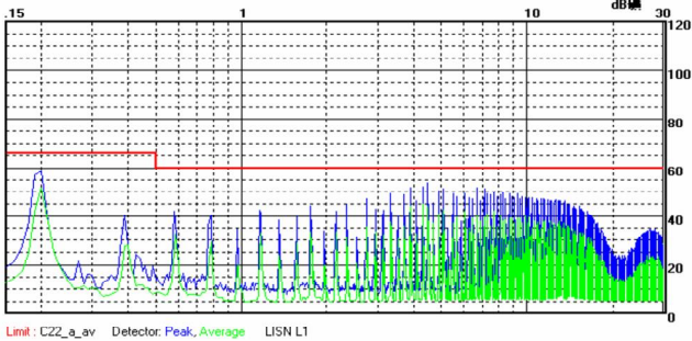
WRA2415P-3WR2 裸机状态下电源正极 (Class A) 测试结果
