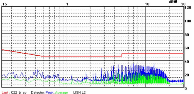
WRA2415P-3WR2 外围状态下电源负极 (Class B) 测试结果
