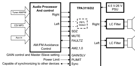
简化应用电路
