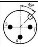
针型 A 键位
