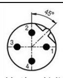
针型 B 键位
