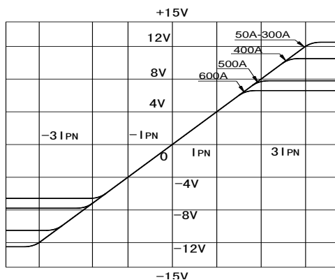
输入电流-输出电压特性
