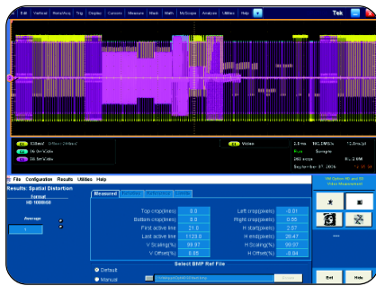
▶ 空间失真显示(选件 SD 和 HD)。
