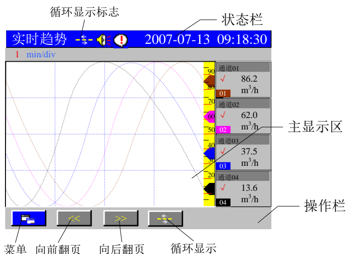
图 6.1 真彩无纸记录仪运行画面区域示意图
