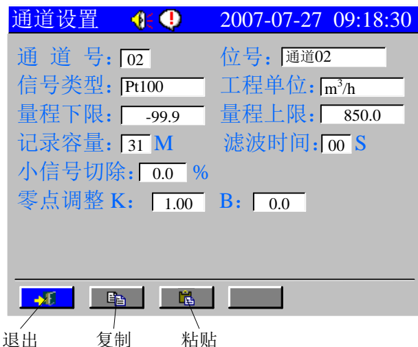
图 5.3 通道设置画面
