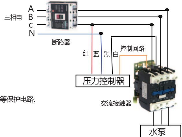
380V三相供电 连接示意图
