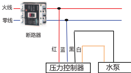
220V供电 负载小于3KW时连接示意图
