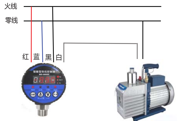
220V供电 负载低于700W时连接示意图
