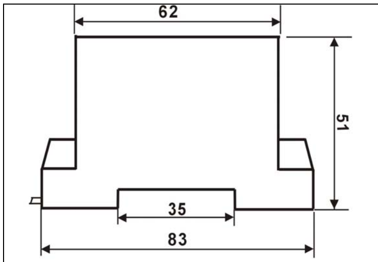
图 4. 产品正视图
