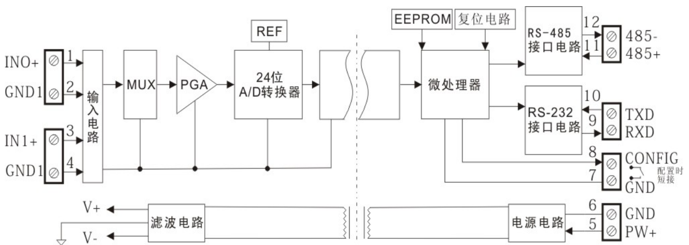
图1. ISO 4021 产品原理框图 请联系：吴茂钦（小吴） 联系电话：18129838285
