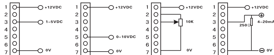
①. 1-5V ②. 0-10V ③. 10K电位器 ④. 4-20ma
