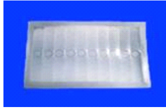
型号: 8719 焦距: 25mm 角度: 90° 距离: 10m 尺寸: 53.5mm×34mm
