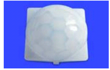
型号: 8002-3 焦距: 12mm 角度: 120° 距离: 10m 尺寸: 直径 24mm
