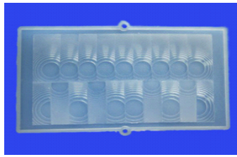
型号: 7704-2B 焦距: 23mm 角度: 110° 距离: 12m 尺寸: 32mm×55mm
