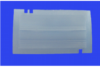
型号: 7809-5 焦距: 21mm 角度: 90° 距离: 9m 尺寸: 43mm×24.5mm
