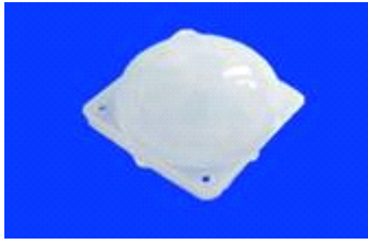
型号: 8002-1 焦距: 10.5mm 角度: 100° 距离: 5m 尺寸: 直径 23mm
