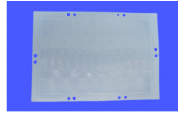
型号: 614230 焦距: 30.5mm 角度: 距离: 尺寸: 60.9mm×42.5mm
