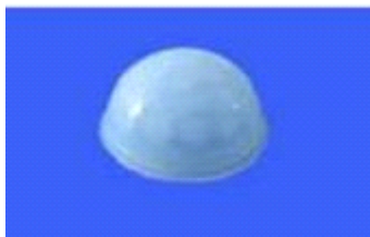
型号: 8005-1 焦距: 10.5mm 角度: 100° 距离: 6m 尺寸: 直径 22.8mm 高 12.4mm
