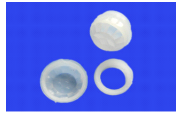
型号: 8120 焦距: 6mm 角度: 120° 距离: 5m 尺寸: 直径 12.7mm
