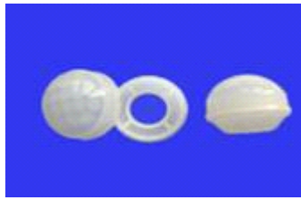
型号: 8090 焦距: 9mm 角度: 120° 距离: 8m 尺寸: 直径 17.8mm 高 14mm
