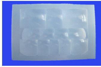
型号: 7601-15 焦距: 21.7mm 角度: 110° 距离: 27m 尺寸: 72.5mm×52mm
