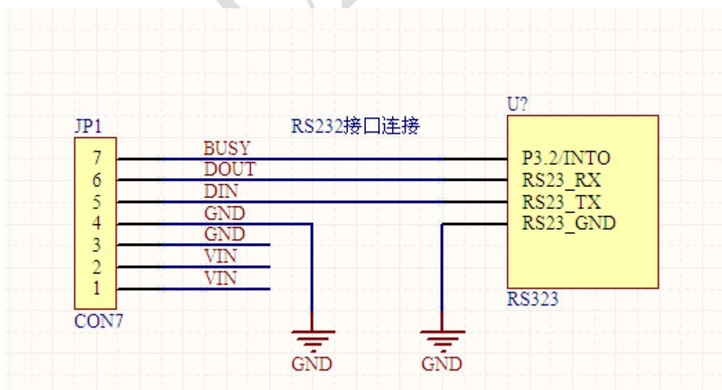
图：RS232 接口连接
