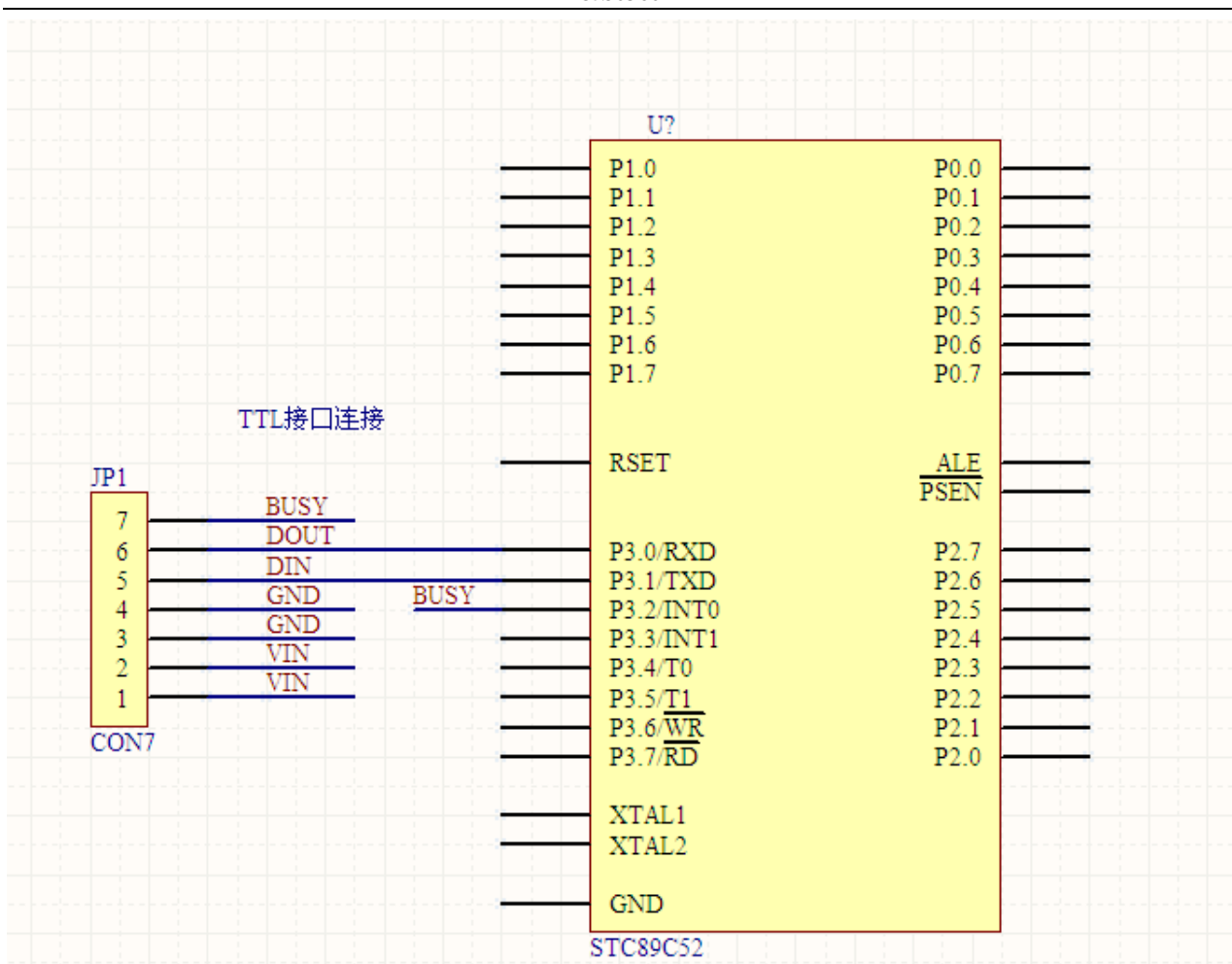
图：TTL 接口连接
