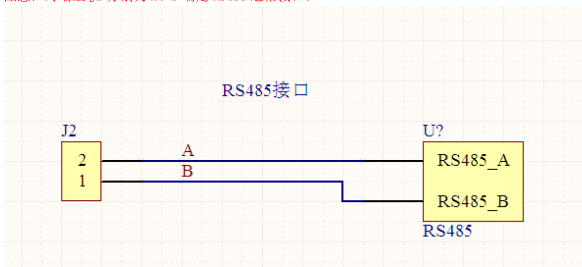
图：RS485 接口连接
