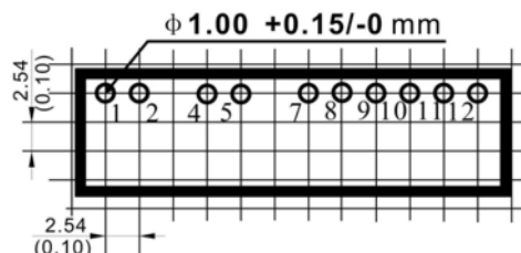
SIP 12 Pin 封装 PCB布板尺寸
