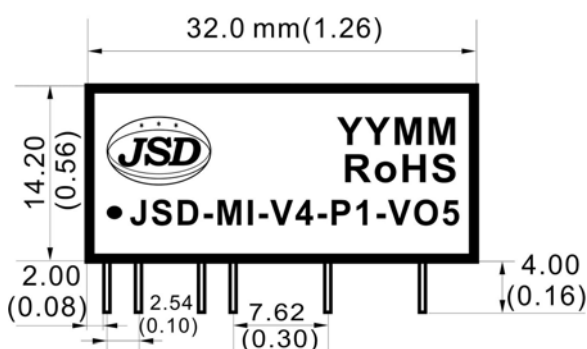
电压输入/电压输出 (V/V隔离)
