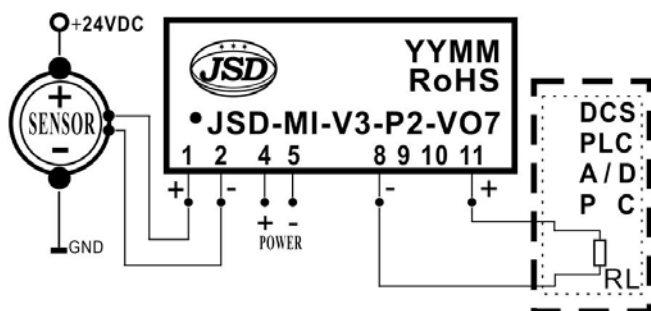
电压输入/电压输出 (V/V隔离)
