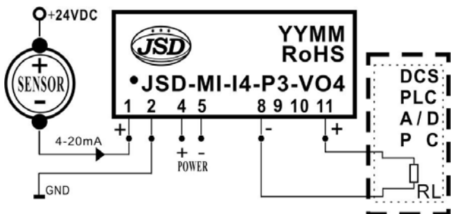
电流输入/电压输出 (I/V转换)
