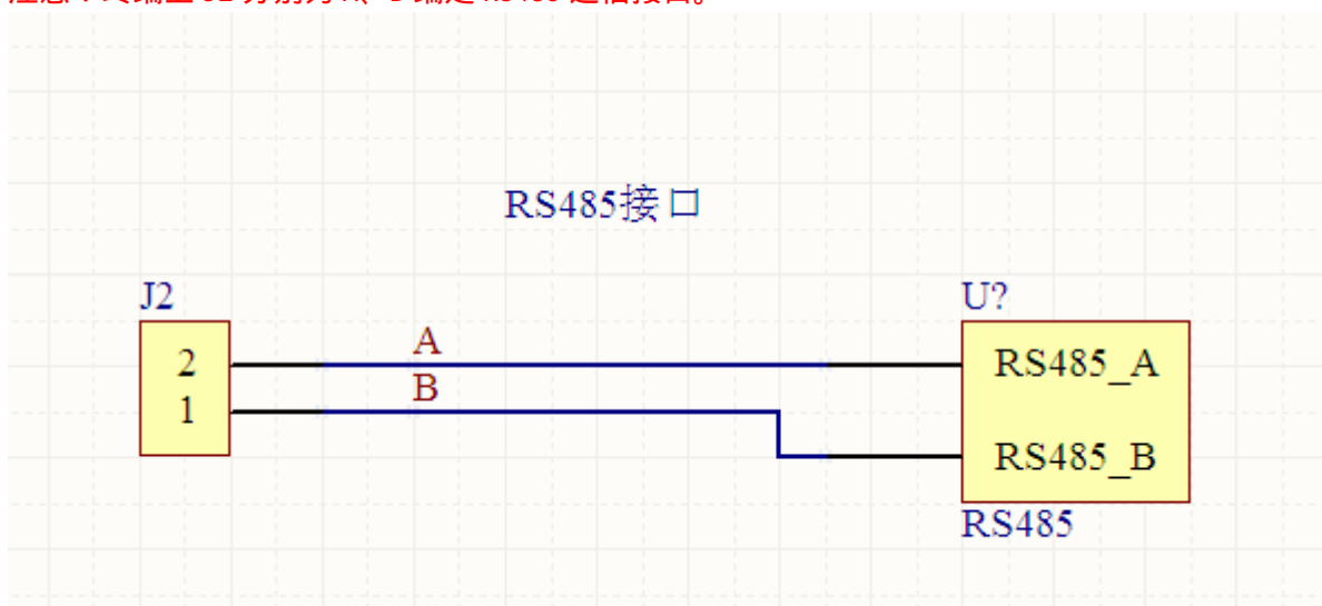
图：RS485 接口连接
