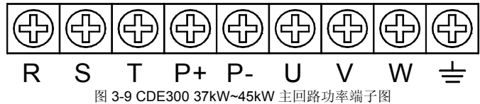
图 3-9 CDE300 37kW~45kW 主回路功率端子图
