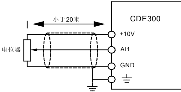
图 3-15 模拟输入端子接线图 1
