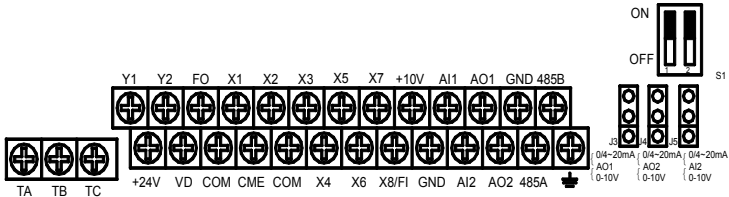
图 3-14 控制端子布局图
