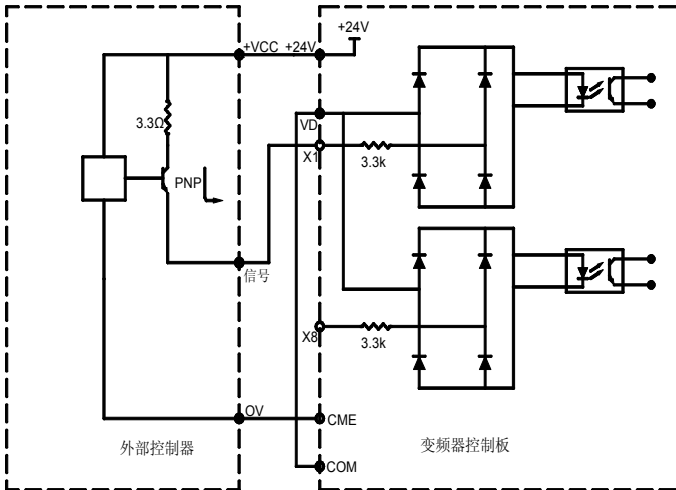
图 3-20 漏极接线方式
