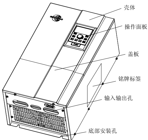
图 2-4 CDE300 18.5kW~132kW 外型图
