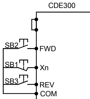
图6-6 三线式运行模式1
