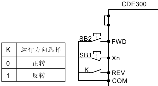
图6-7 三线式运行模式2
