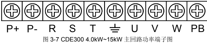
图 3-7 CDE300 4.0kW~15kW 主回路功率端子图
