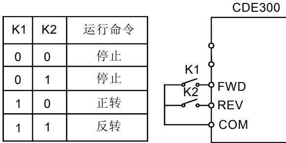
图6-5 两线式运行模式2
