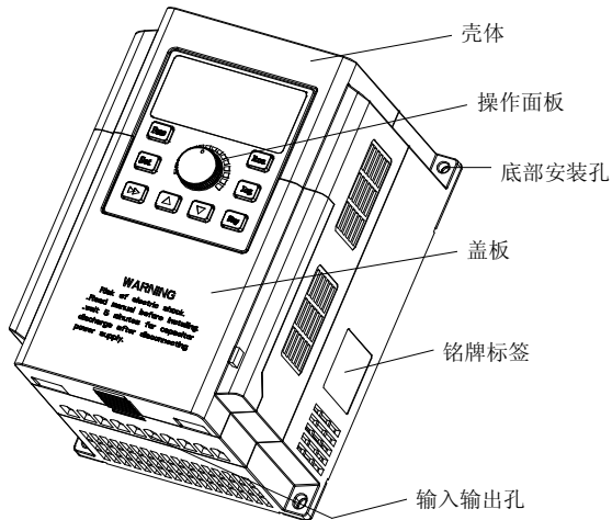
图 2-3 CDE300 15kW 及以下外型图
