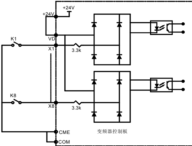
图 3-17 干接点共阴极接线方式
