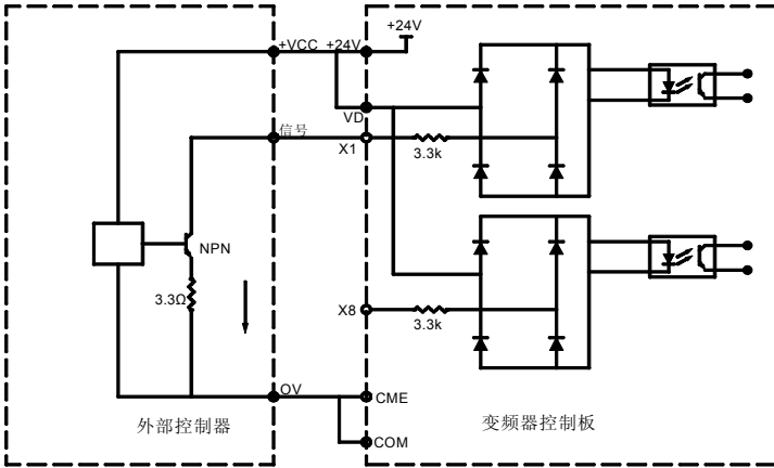
图 3-19 源极接线方式
