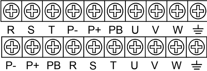
图 3-6 CDE300 0.7kW~2.2kW 主回路功率端子图
