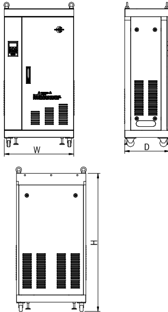
图 2-8 CDE300 160kW 及以上安装尺寸
