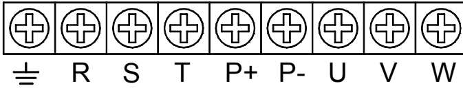
图 3-12 CDE300 160kW~280kW 主回路功率端子图
