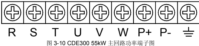
图 3-10 CDE300 55kW 主回路功率端子图
