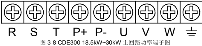
图 3-8 CDE300 18.5kW~30kW 主回路功率端子图
