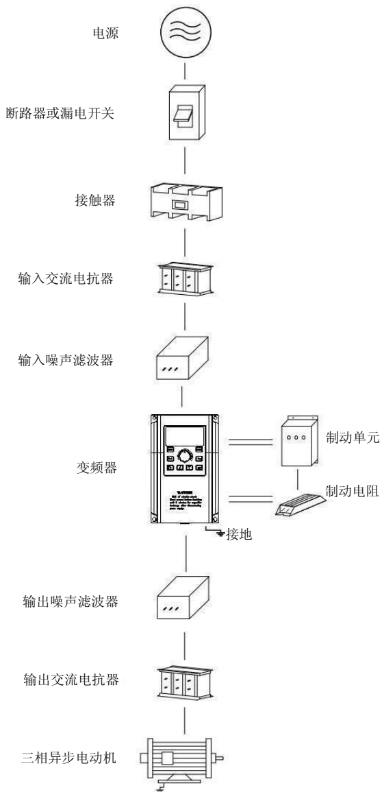
图 3-4 与外围设备的连接图
