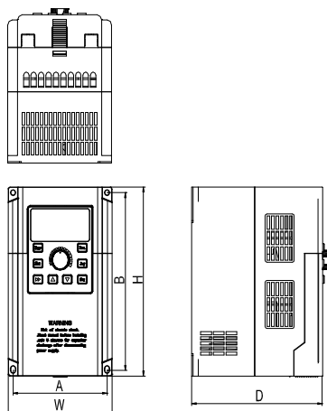
图 2-6 CDE300 15kW 及以下安装尺寸
