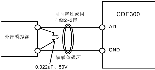
图 3-16 模拟输入端子接线图 2
