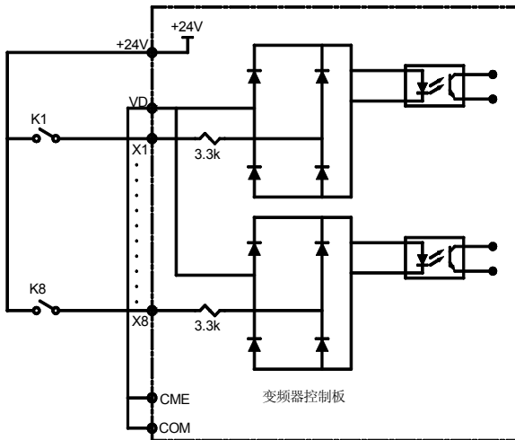
图 3-18 干接点共阳极接线方式
