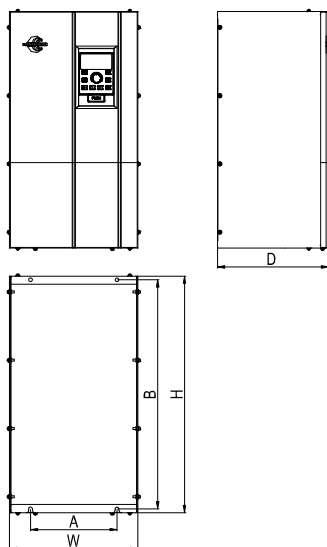
图 2-7 CDE300 18.5kW~132kW 安装尺寸
