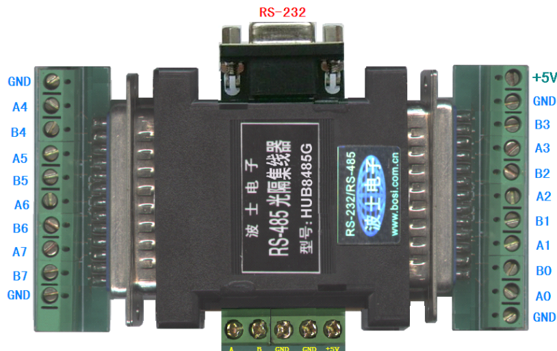
图为波仕新一代 HUB8485G
