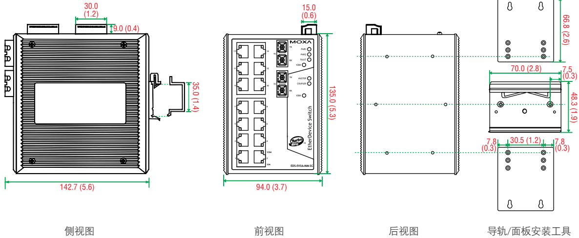
侧视图
