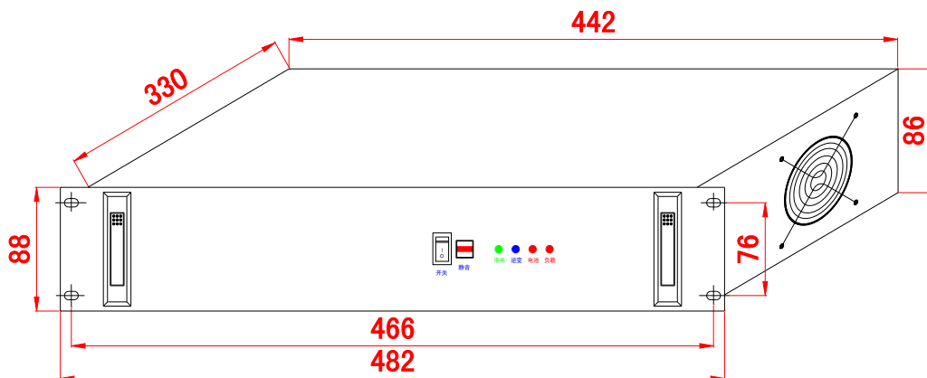
C 型机箱：1KVA、2KVA 逆变电源（LED型）外形机械尺寸图 单位：mm 误差：±0.5mm
