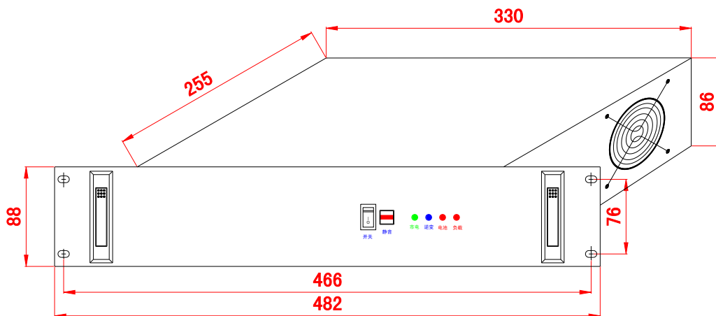
B 型机箱：500VA 逆变电源（LED型）外形机械尺寸图 单位：mm 误差：±0.5 mm
