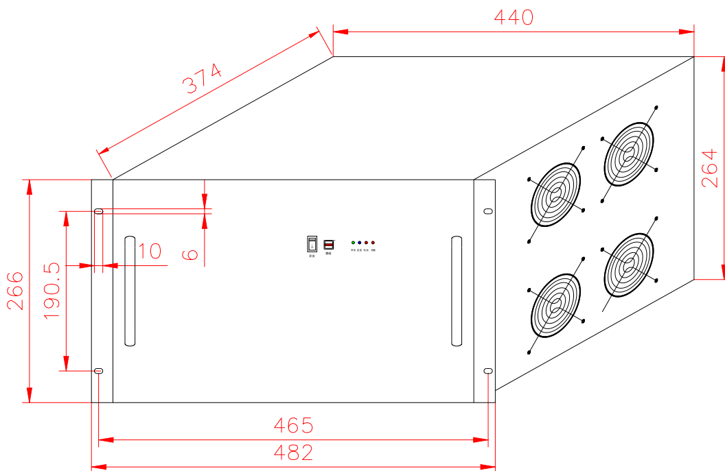
M型机箱：8KVA-10KVA 逆变电源（LCD）外形机械尺寸图 单位：mm 误差：±5%
