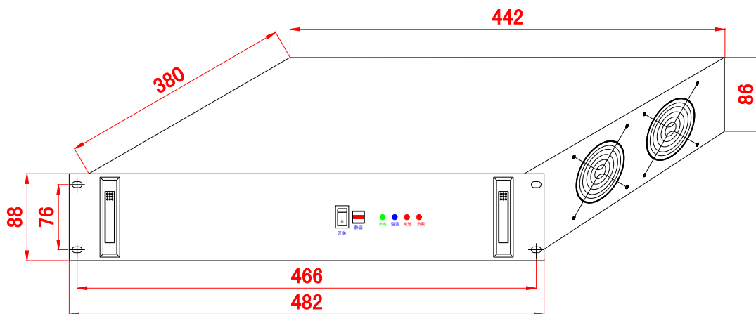
G型机箱：3KVA-6KVA 逆变电源（LED型）外形机械尺寸图 单位：mm 误差：±5%
