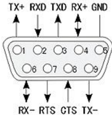
RS232 通讯端口
