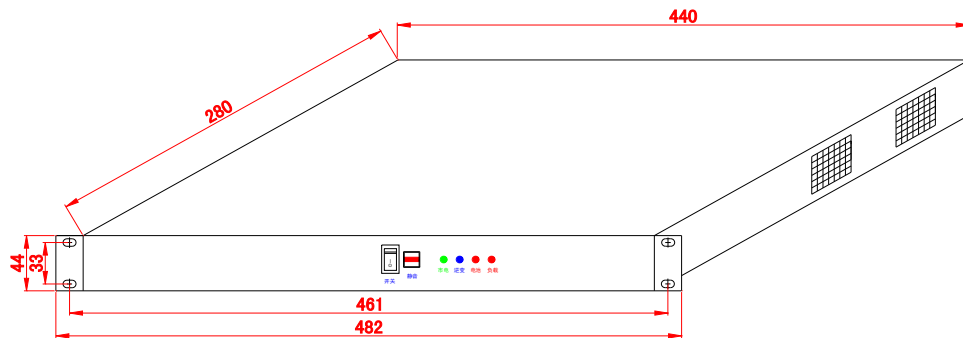
A 型机箱：500VA 逆变电源（1U高）外形机械尺寸图 单位：mm 误差：±0.5%
