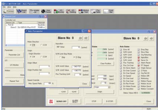
Axis Parameter Set up
