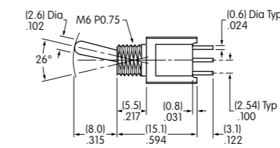
面板密封·双极
