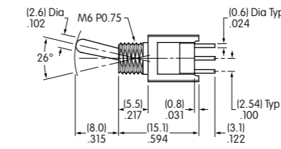
面板密封·单极
