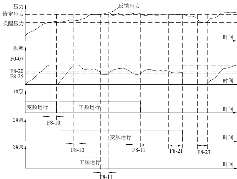
系统运行时序图
