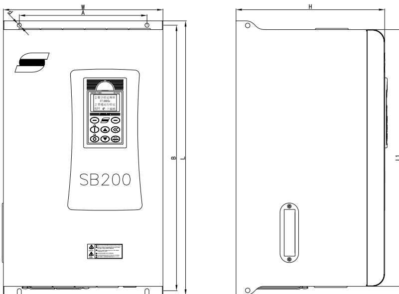
SB200-30T4及以上机型外形图
