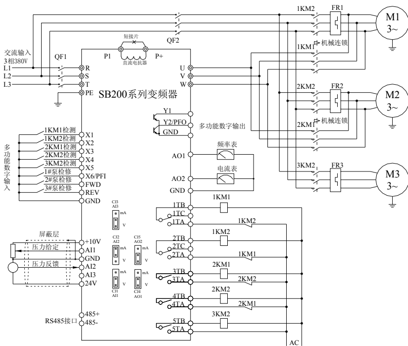
变频循环投切一控二和一台辅助泵的应用图
