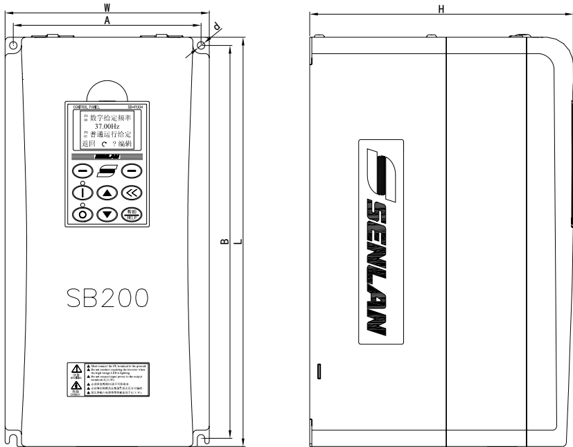
SB200-1.5T4~5.5T4机型外形图（可用标准DIN导轨安装）
