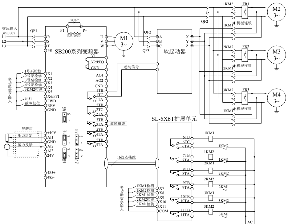
变频器加软启动器恒压供水应用图
