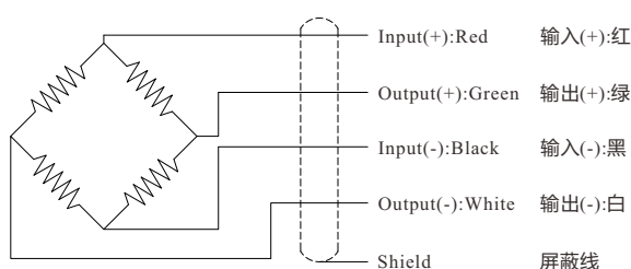
Wiring Diagram/接线图
