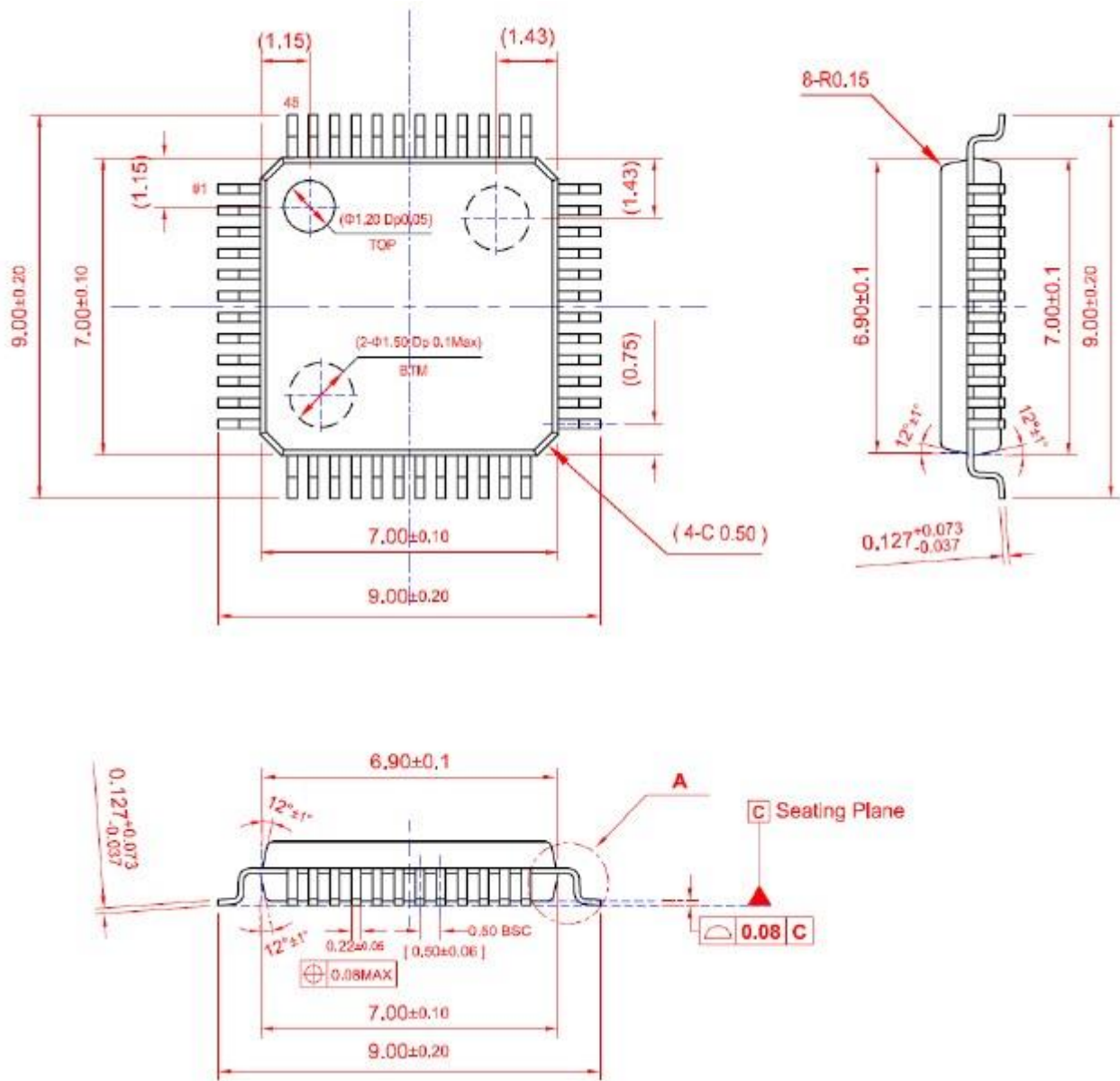
图 25 封装描述
