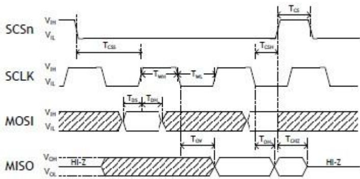
图 23 SPI 时钟
