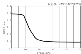
力矩曲线图
