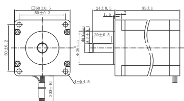
尺寸图
