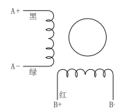
接线图
