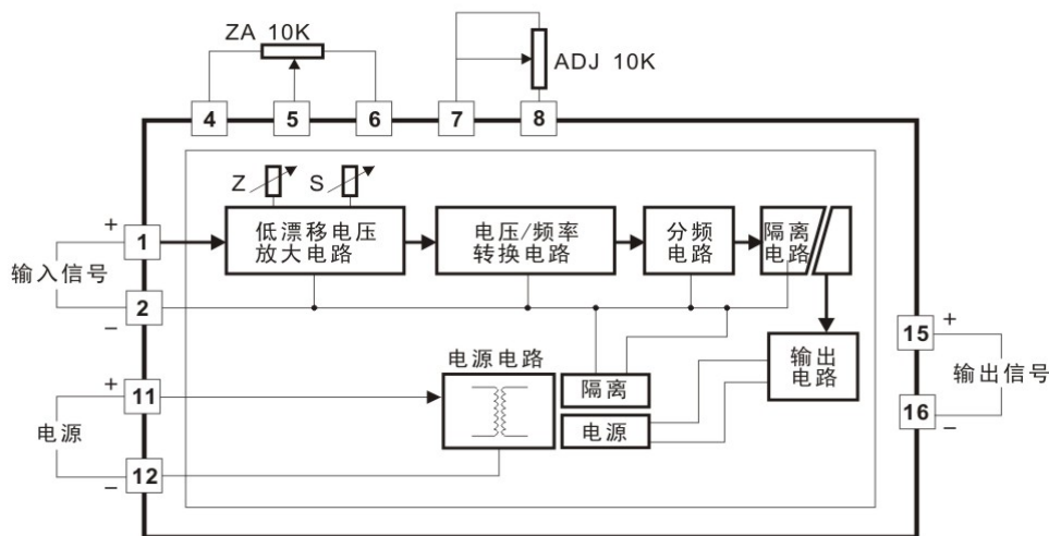
ISO-U(A)-P-F 系列隔离变送器原理框图
