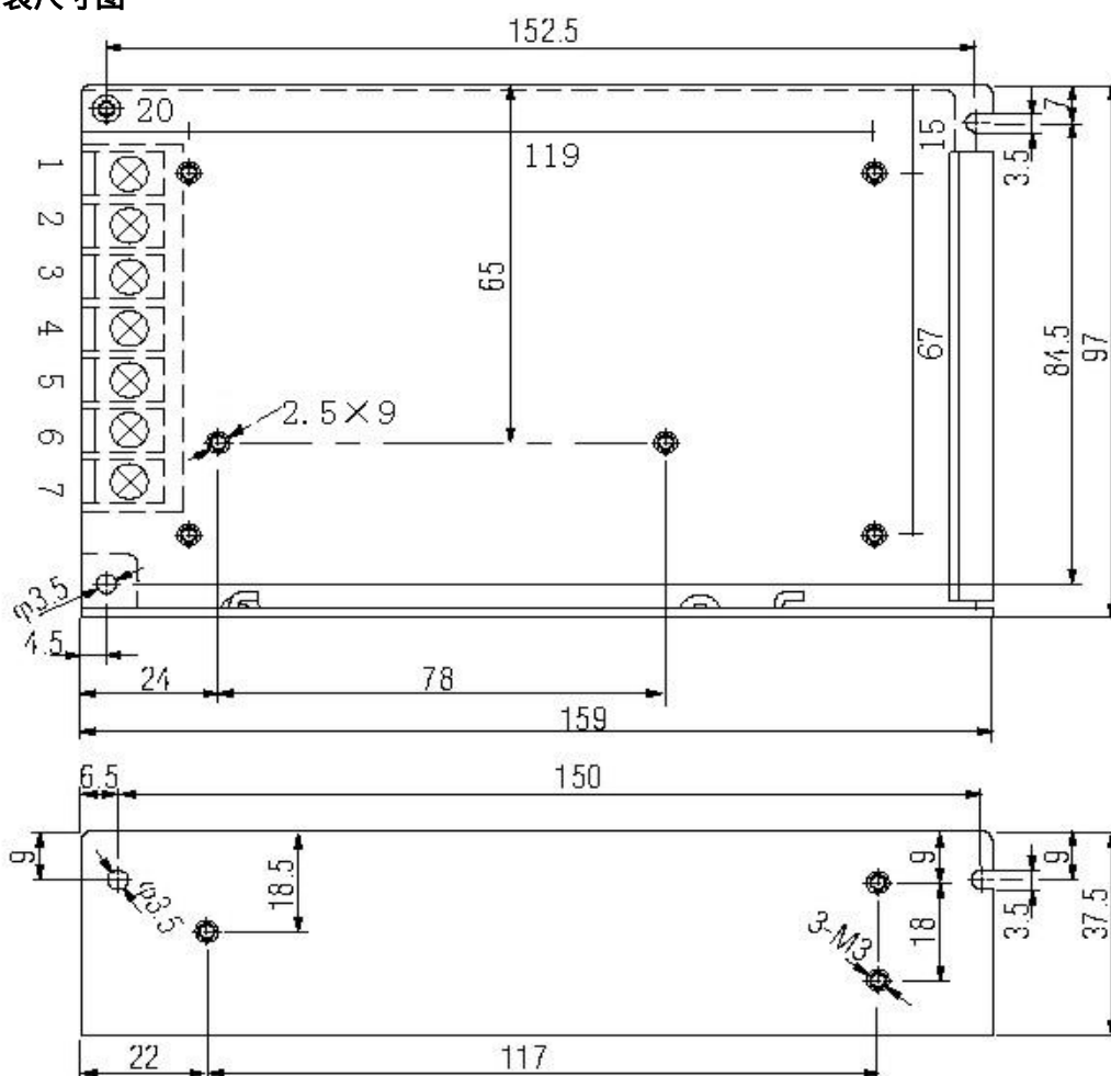
安装尺寸图
