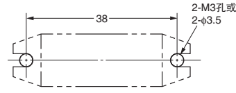
安装孔加工尺寸 (BOTTOM VIEW) 尺寸公差为±0.1mm
