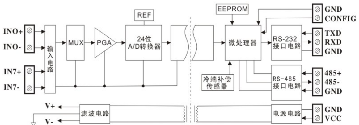
图1 SYAD08T 产品原理及外接端子框图
