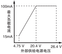
[ 输出电路·源型 ]
