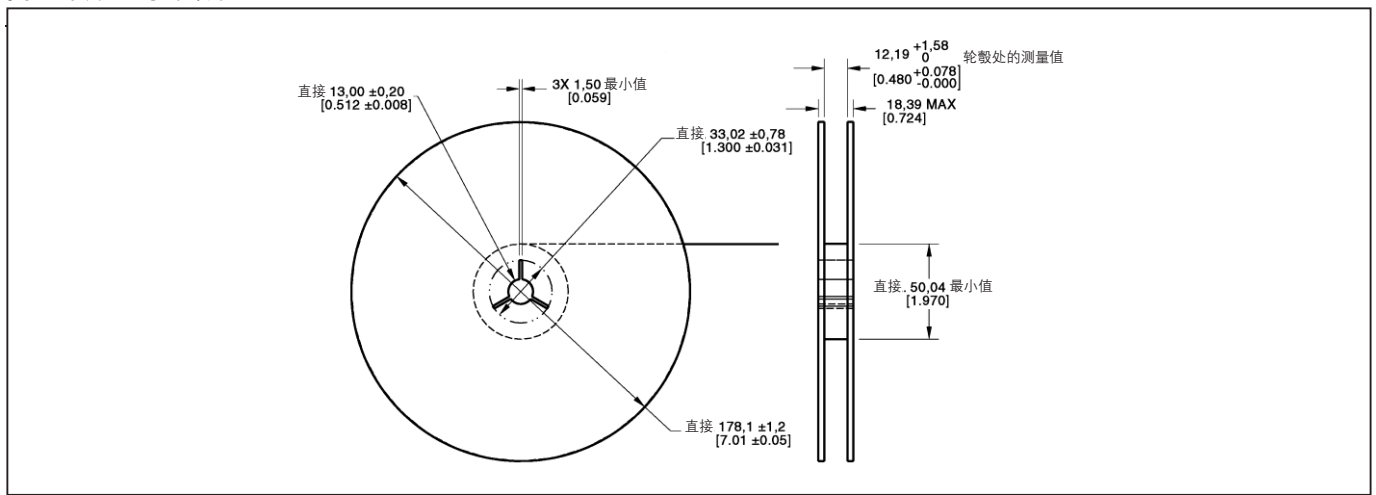
图3: 安装尺寸 (续)
