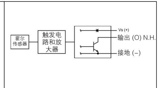
图3: 灌电流输出框图
