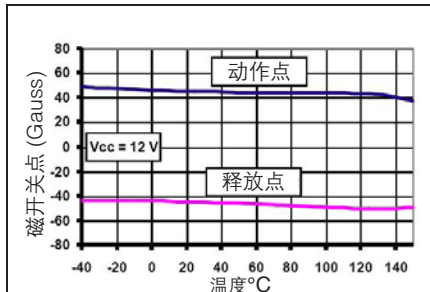
图1: 典型磁特征参数
