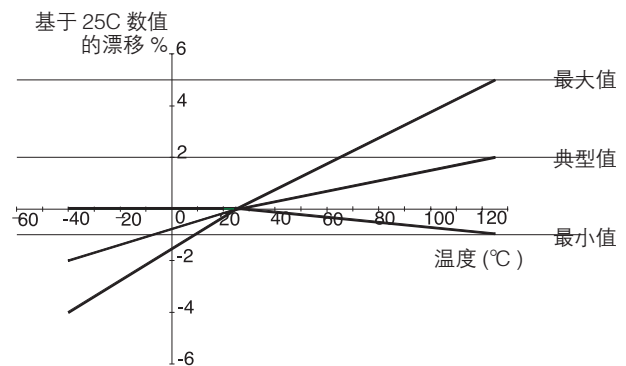
图 2-9: 灵敏度温漂
