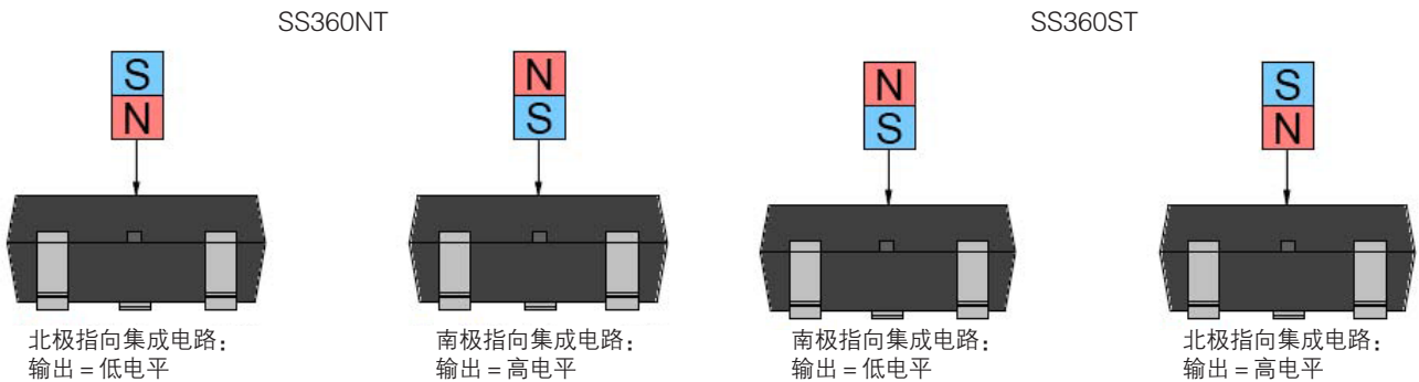
图4：磁性激励
