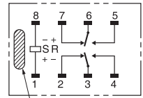
端子配置/内部连接图 (BOTTOM VIEW)
