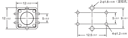
端子配置/内部连接图 (TOP VIEW)
