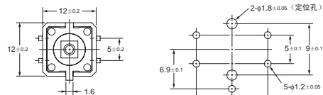
端子配置/内部连接图 (TOP VIEW)
