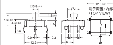
端子配置/内部连接图 (TOP VIEW)
