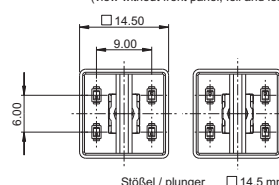
Platzierungsmöglichkeiten der LED's (Ansicht ohne Frontplatte, Folie und Blende) placement options of the LEDs (view without front panel, foil and lens)
